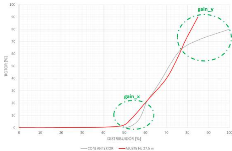
Figura 11 – Resultados de ajuste de conjugação – baixa e alta potência. Fonte: acervo próprio
