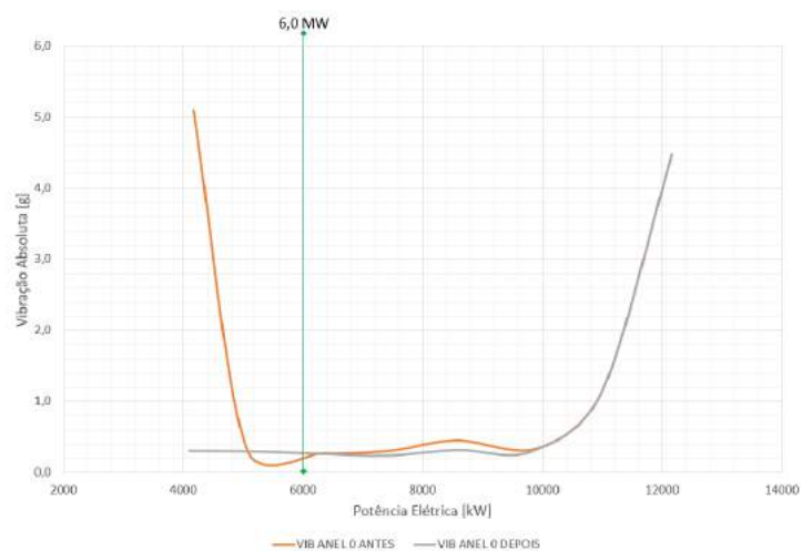
Figura 13 – Resultados de melhorias em vibrações com ajuste de conjugação. Fonte: acervo próprio
