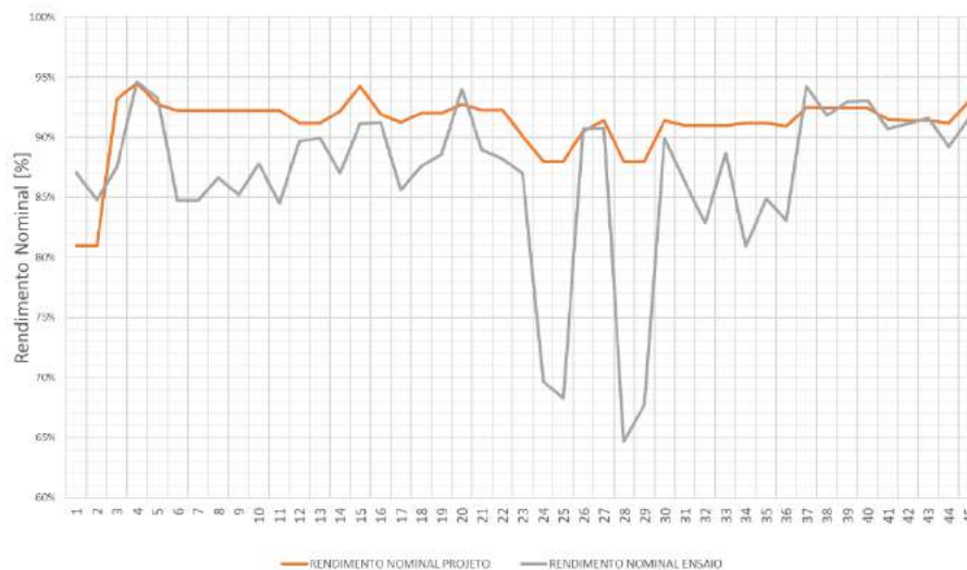
Figura 9 – Levantamento de rendimentos de projeto x rendimento real de diversas usinas e máquinas. Fonte: acervo próprio
